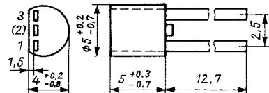
Bild 1: Gehäuseabmessungen und Anschlußbelegung des B 589 N
