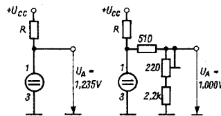
Bild 6: Einfachste Referenzspannungserzeugungsvarianten
