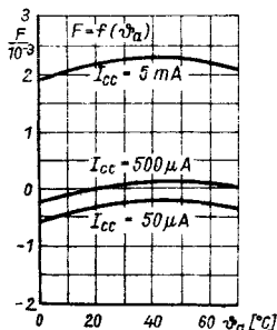
Bild 3: Praktische Abweichung vom linearen TK
