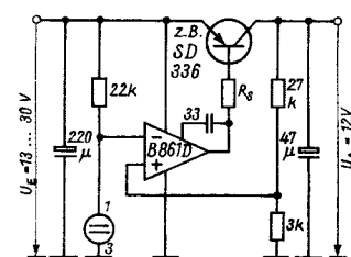
Bild 7: Strombegrenzendes Netzteil
