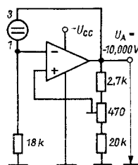
Bild 5: Negative Referenzspannungserzeugung
