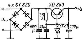
Bild 6: Einsatz des SD 350 als Längstransistor in einem Netzteil mit Spannungsstabilisierungsschaltung
