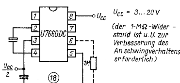
Bild 18: Anwendung des U7660 DC zur exakten Halbierung der anliegenden Betriebsspannung
