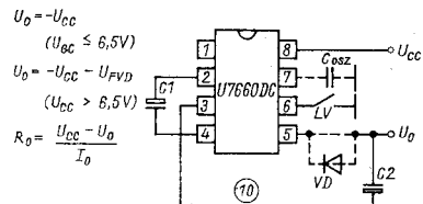
Bild 10: Betriebsspannungsinverter für negative Ausgangsspannung. Zur Beschriftung siehe Applikationshinweise und Kennlinien.
