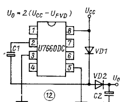
Bild 12: Beschriftung zur Verdopplung der Betriebsspannung
